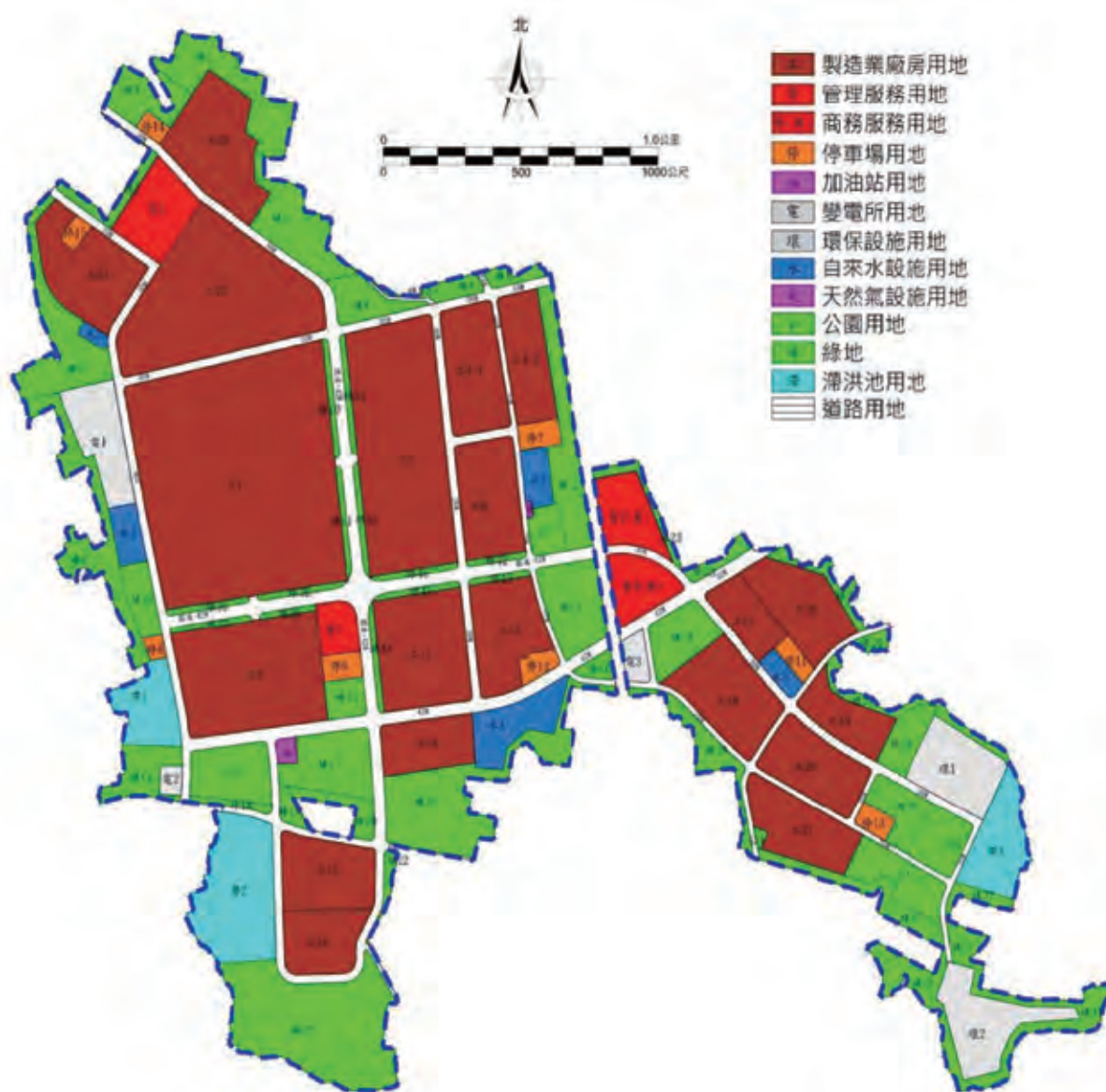
圖 3 高雄園區土地使用計畫示意圖
