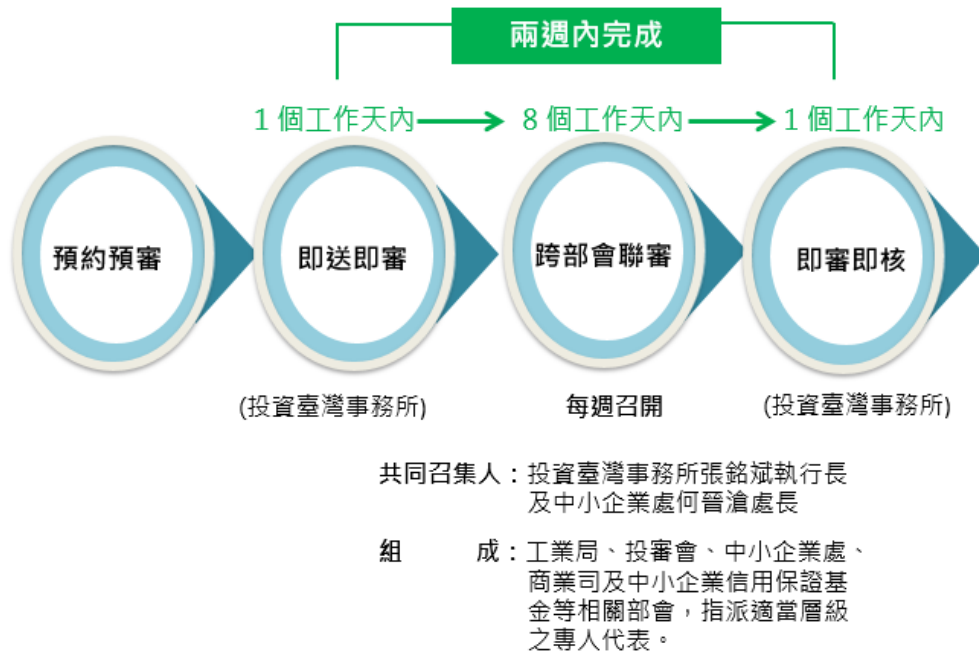
圖 3 審核流程
